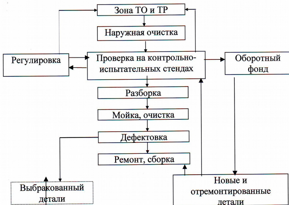
Схема технологического процесса цеха ремонта топливной аппаратуры
